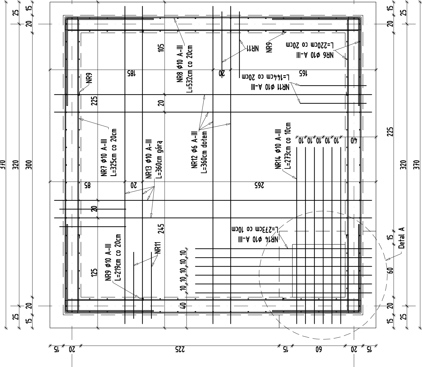
Poz. 2. i 3. Ściany i płyta dolna pom. tech.
